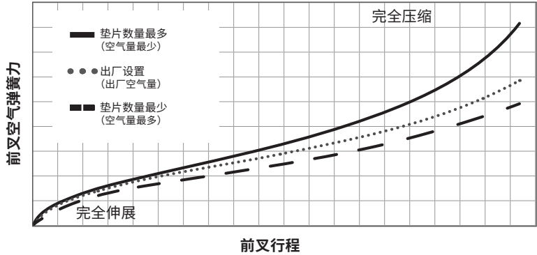
典型的空气弹簧曲线
