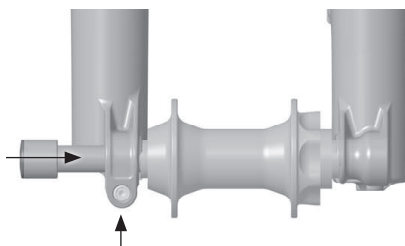
Perno de aperto em pinça (Pinch bolt)
